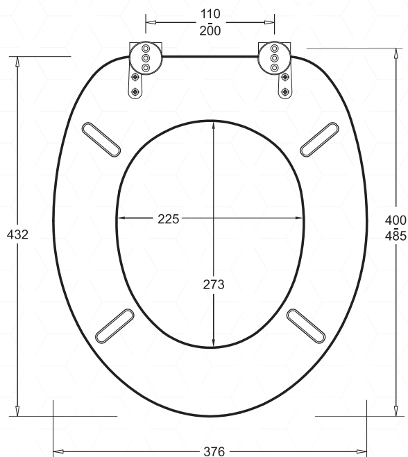
DIMENSIONS
